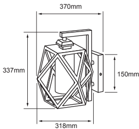
ALTER III 60FTL3434MVCA ■ Negro/Ambar POTENCIA: 60 W máx. LÁMPARA SUGERIDA: Filamento LED VOLTS: 100-240 V ~ Tipo de lámpara: Opcional (No incluida) Tipo de base: E27
